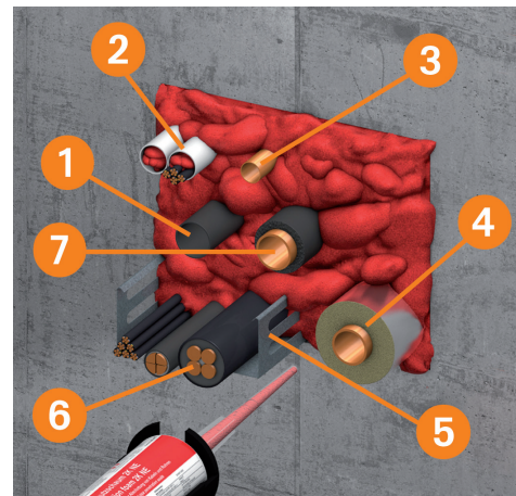
Montageschema
